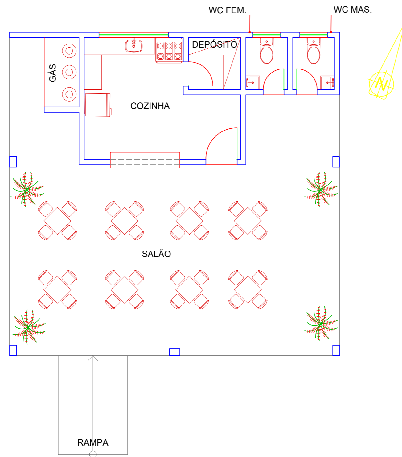
PLANTA DE LAYOUT ESCALA: 1/50
