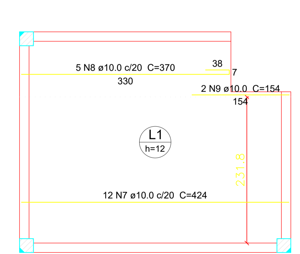
ARMADURAS POSITIVAS
